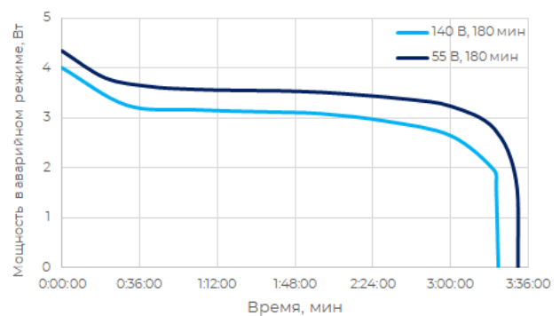
Рис. 4 - Зависимость мощности в аварийном режиме от времени разряда (на max и min нагрузке)
