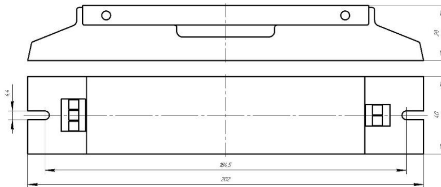
Рисунок 1 – Габаритные размеры Star 50-350T Lite M, Star 60-700T Lite
