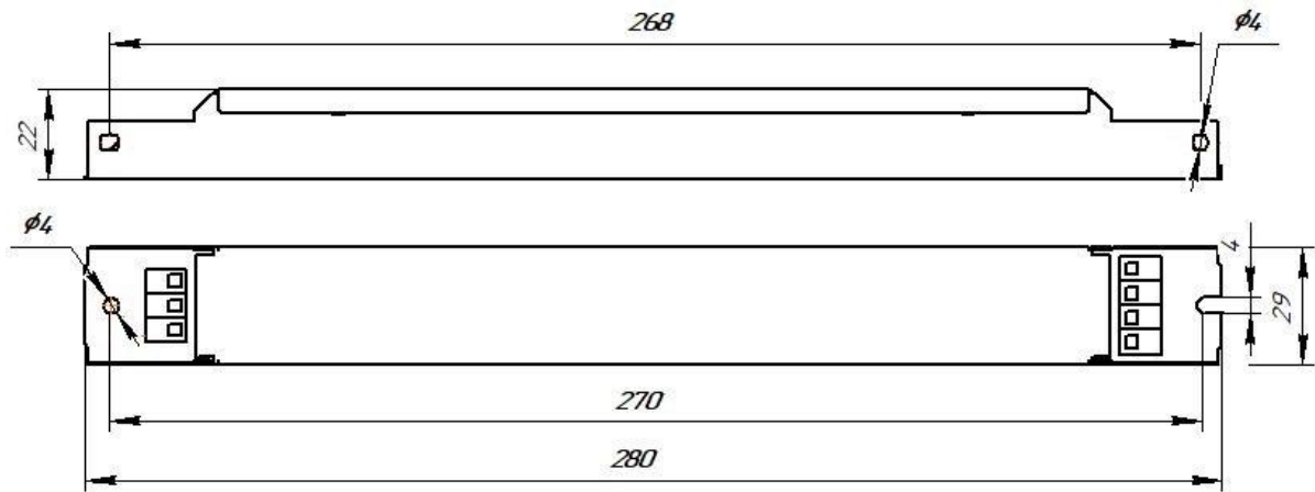
Рисунок 2 – Габаритные размеры Star 80-700T Lite
