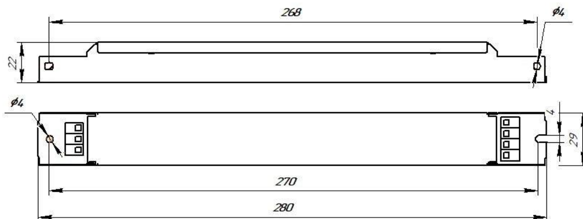
Рисунок 1 – Габаритные размеры Star 35-400...700TD Elegant
