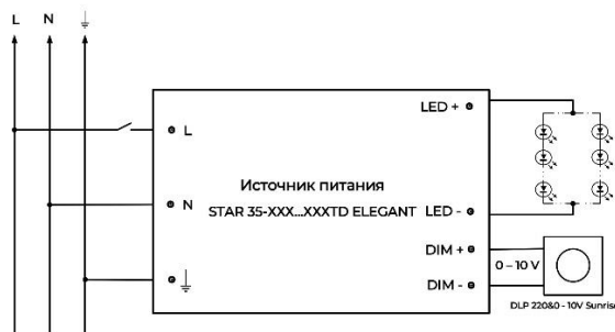
Рисунок 2 – Схема подключения
