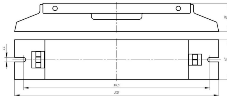
Рисунок 1 – Габаритные размеры Star 50-300/350TR Flagman
