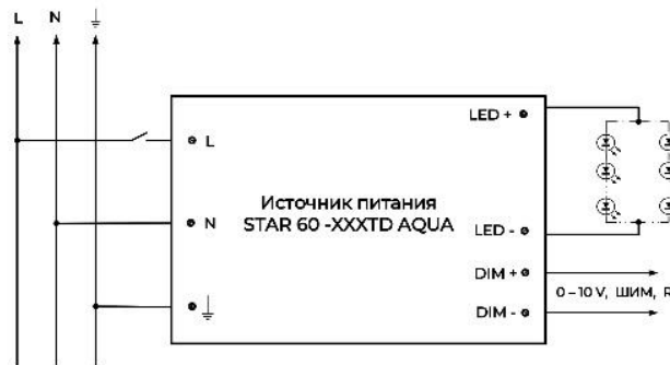
Рисунок 2 – Схема подключения
