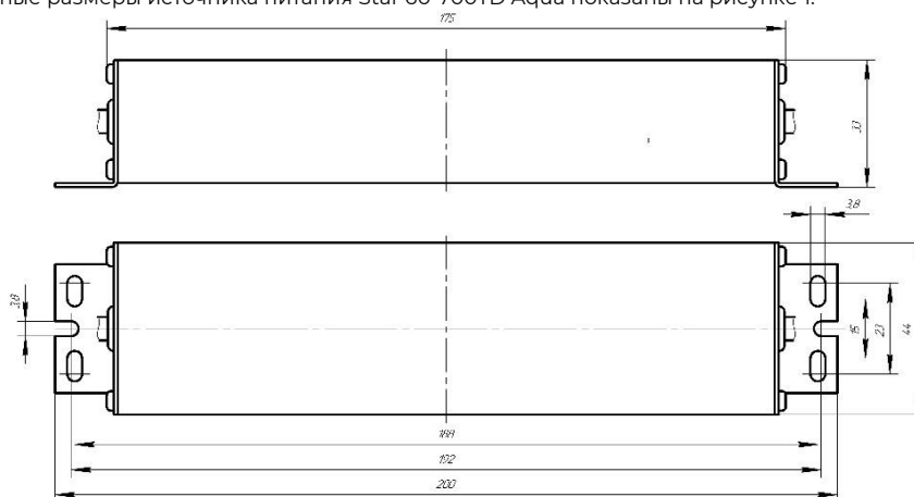
Рисунок 1 – Габаритные размеры Star 60-700TD Aqua
