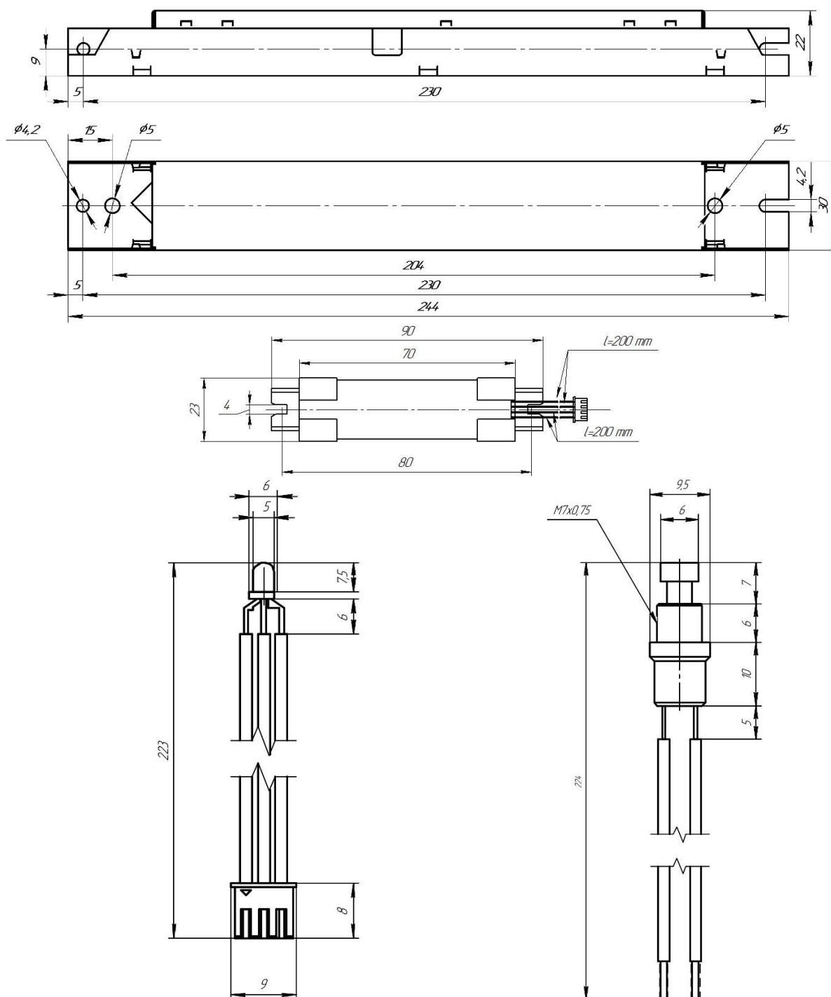
Рисунок 1 – Габаритные размеры источника STAR 20-350T-LS1 Neuron
